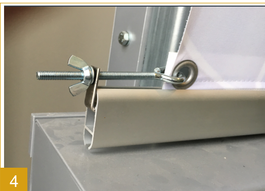
4 Detalje af sidestrammer.
