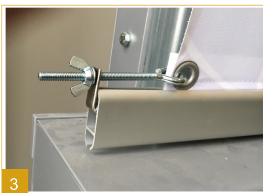
Detalje af sidestrammer.
